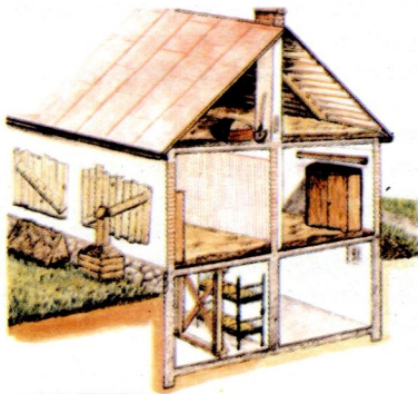
Radioaktívbiztos óvóhely a családi ház alagsorában
